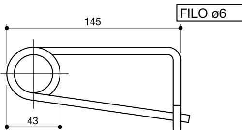
SPILLONE di sicurezza 6 x 145
