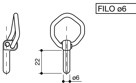
SPINOTTO a scatto per erpice
