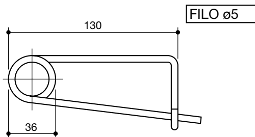
SPILLONE di sicurezza 5 x 130
